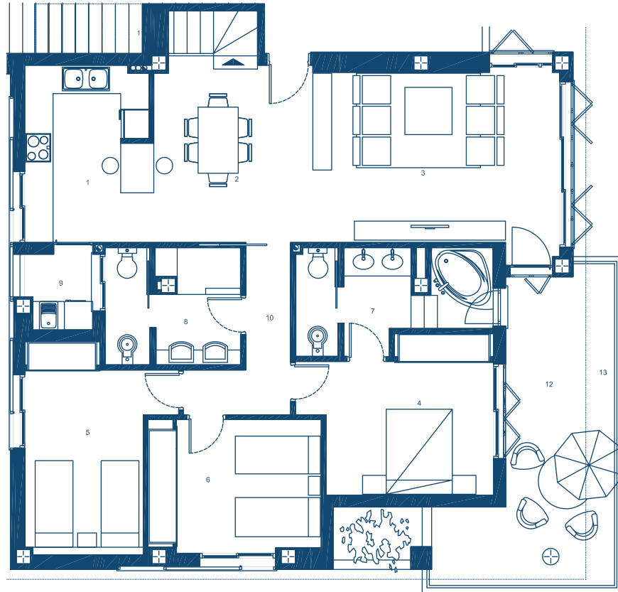
PLANTA SEGUNDA / SECOND FLOOR
